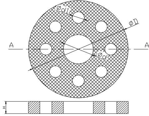
A-A' KESİTİ
